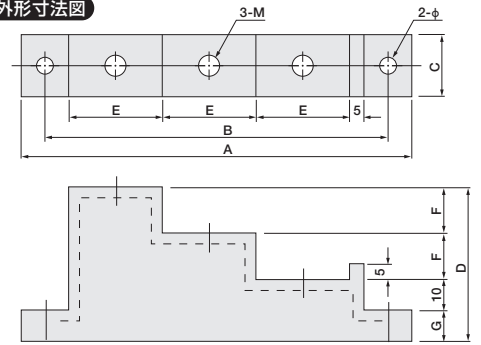
▼外形寸法図
