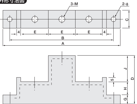
▼外形寸法図
