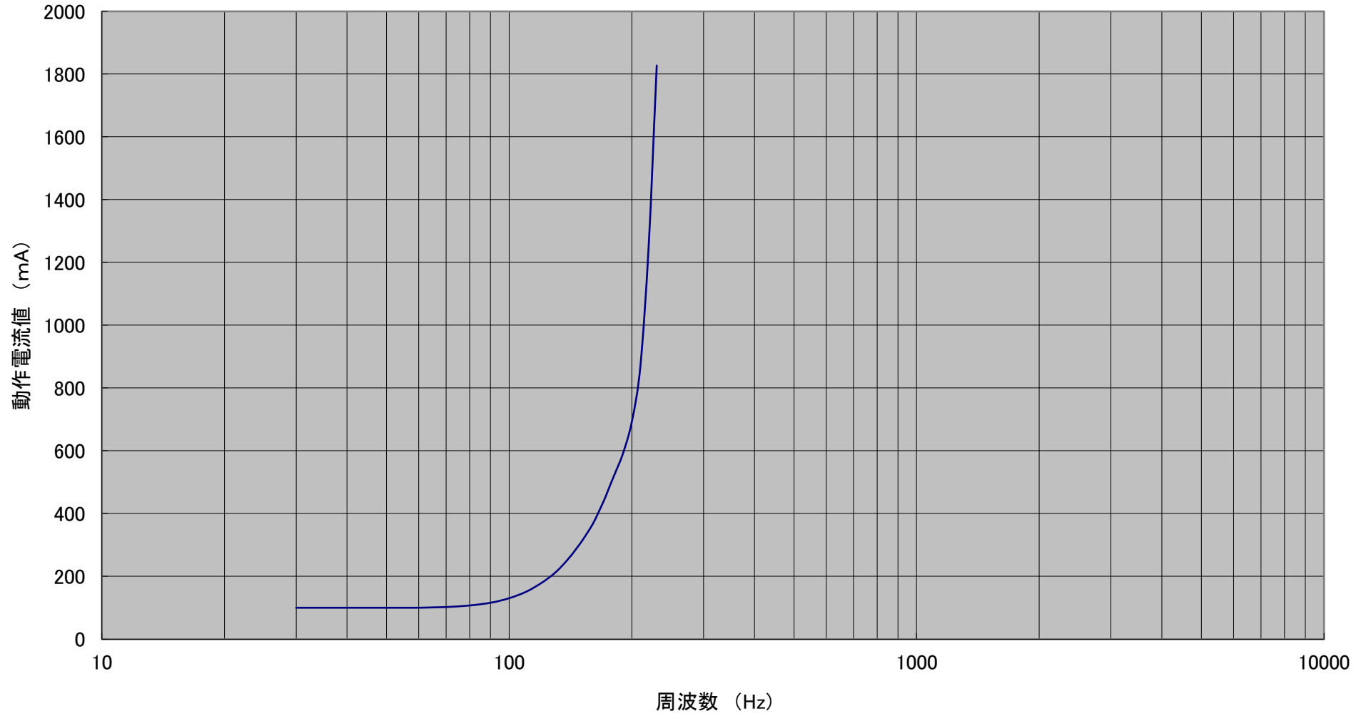
漏電継電器 LL-50BK□ の周波数特性 50Hz 100mA整定
