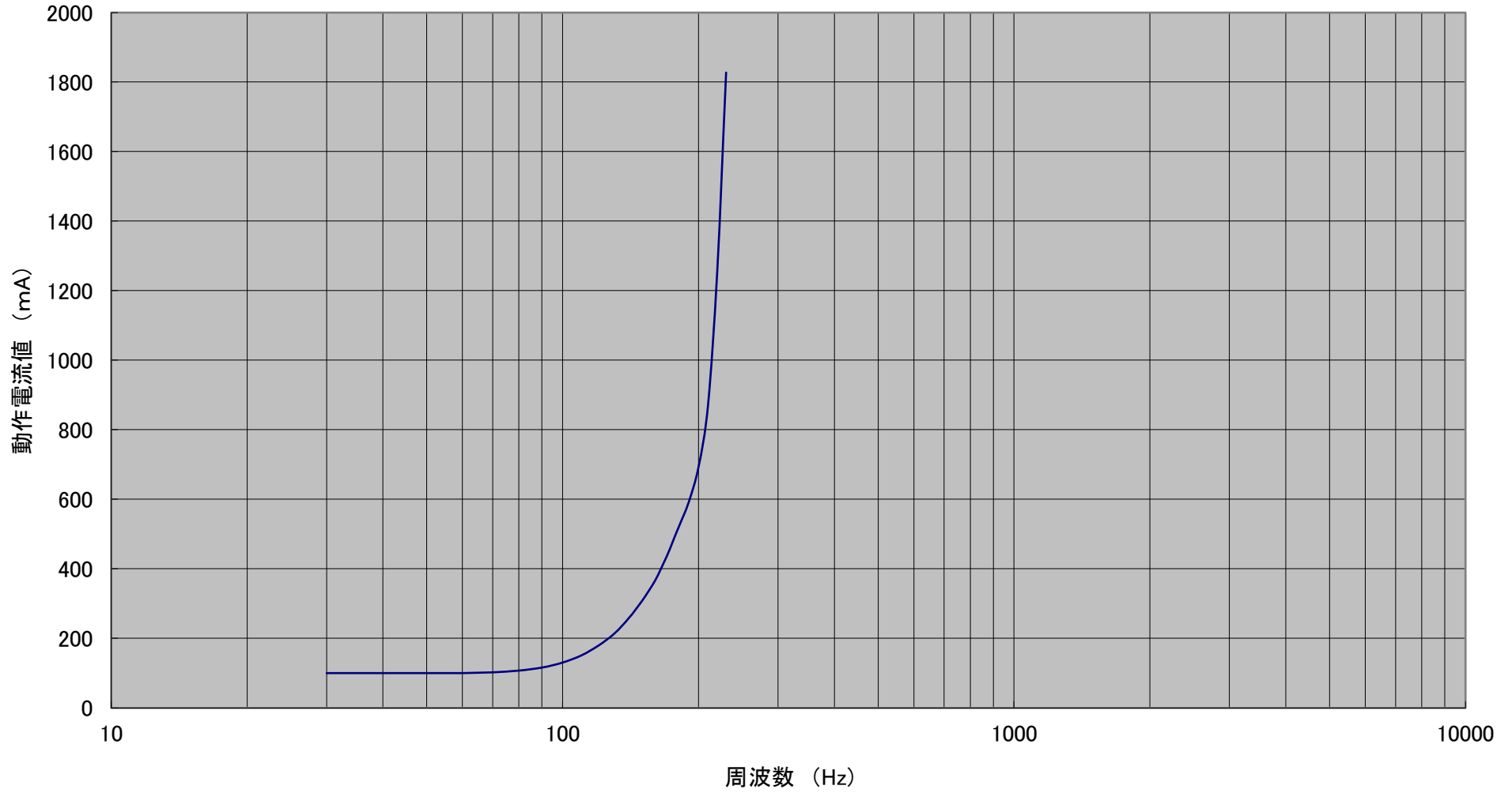
漏電継電器 UP-50BK□ の周波数特性 50Hz 100mA整定
