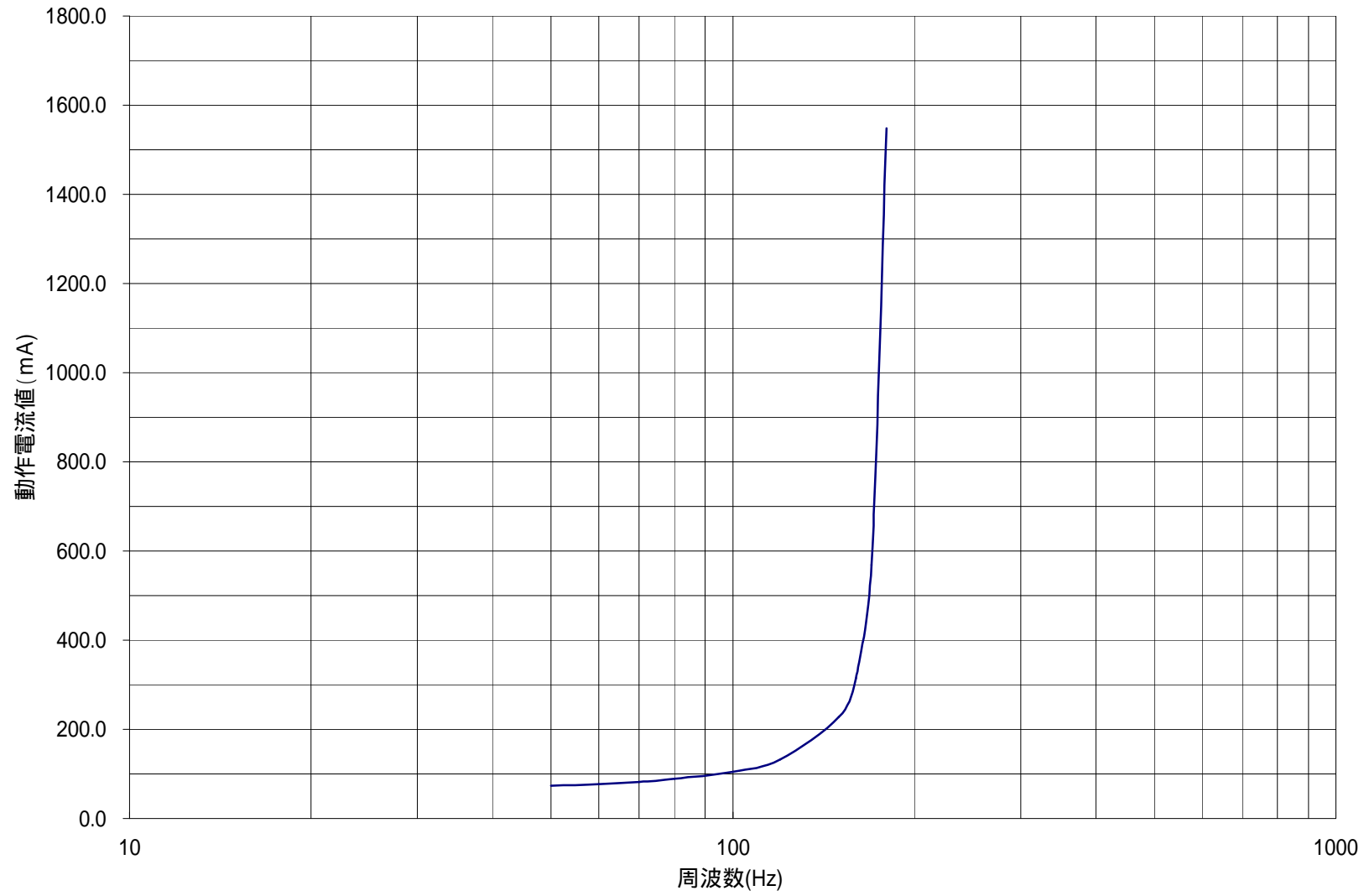
LL-30D2 LL-30Mの周波数特性 整定値100mA
