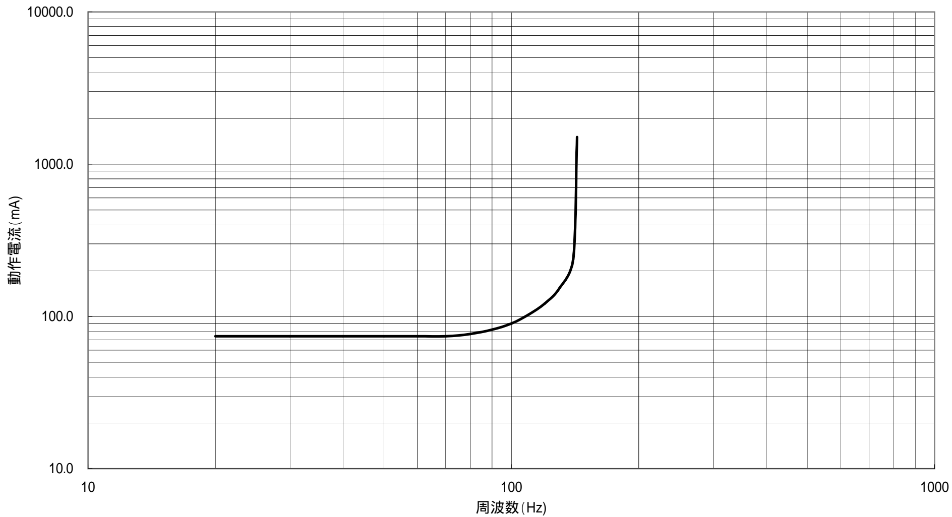
LL-30MP 周波数特性 整定値100mA 50Hz
