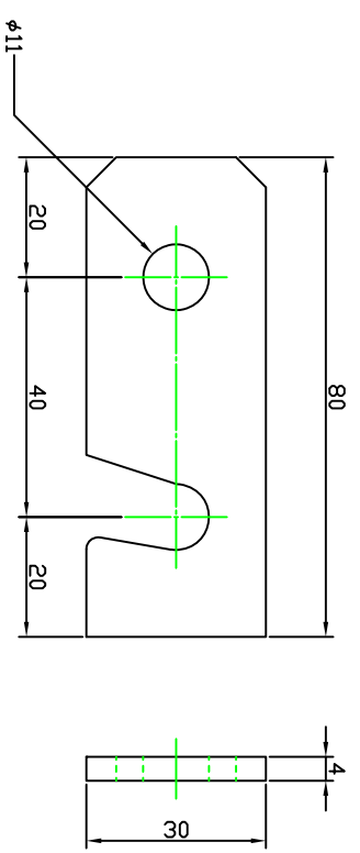
可動バー
