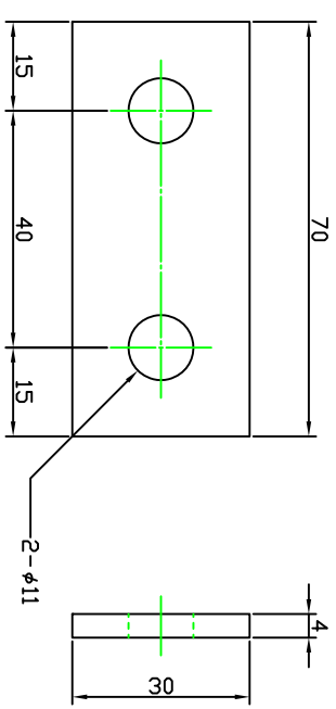
固定バー
