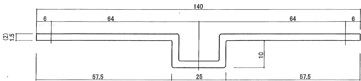
SB-2 (SB-2K)
