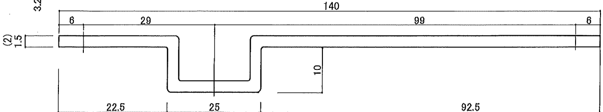
RTB-2 (RTB-2K)
