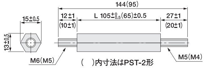
▼外形寸法図
