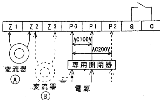
LGA-6F (壁掛形)
