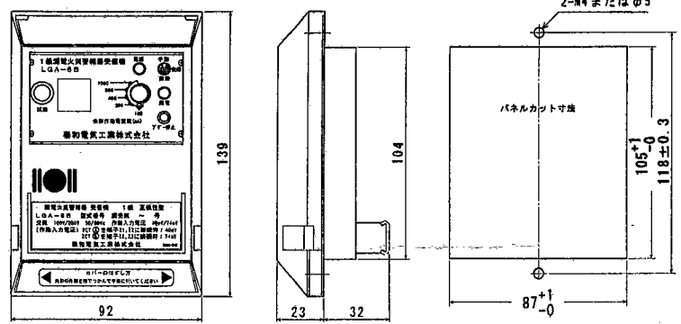
LGA-6B (埋込形)
