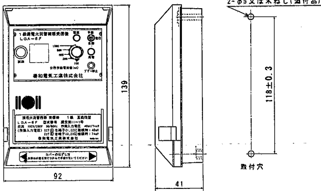
LGA-6F (壁掛形)
