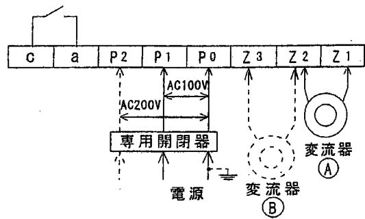
LGA-6B (埋込形)
