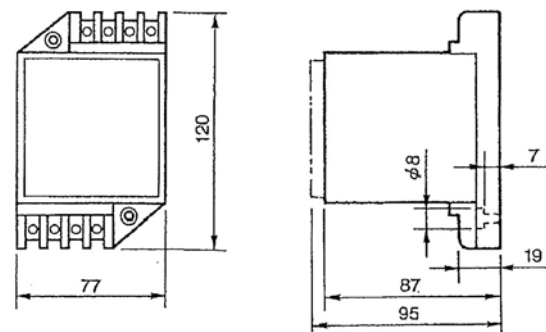
図2 外形寸法図
