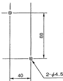
図1 パネル穴あけ寸法
