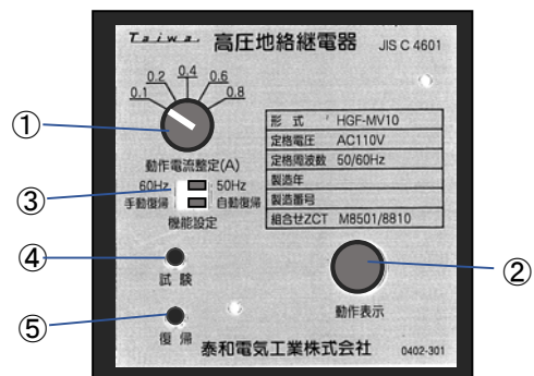
図5 高圧地絡継電器 正面図
