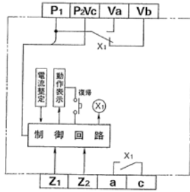
図3 HGF—MV10 端子配列
