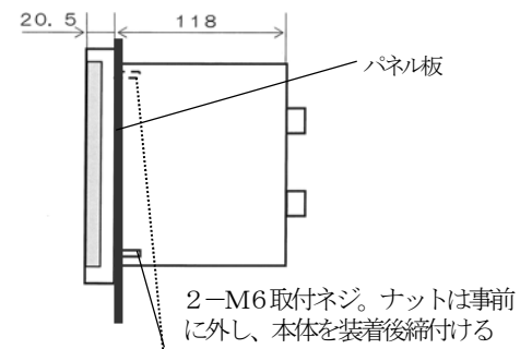
図2 取付け状態尾図
