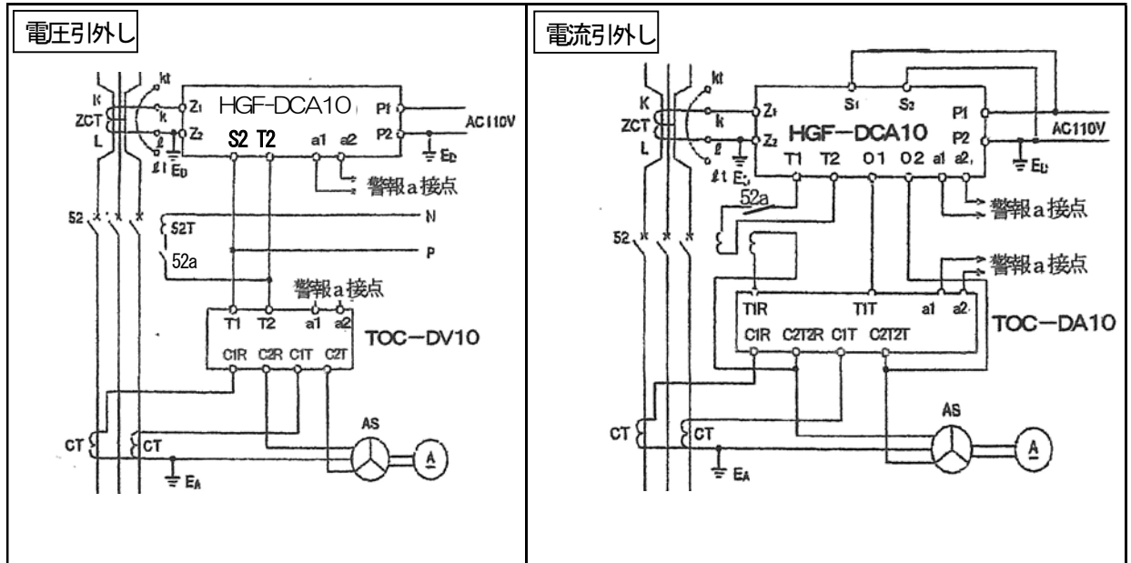
図4 外部接続図例
