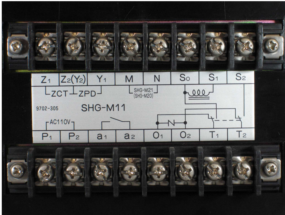
SHG - M11 端子配列
