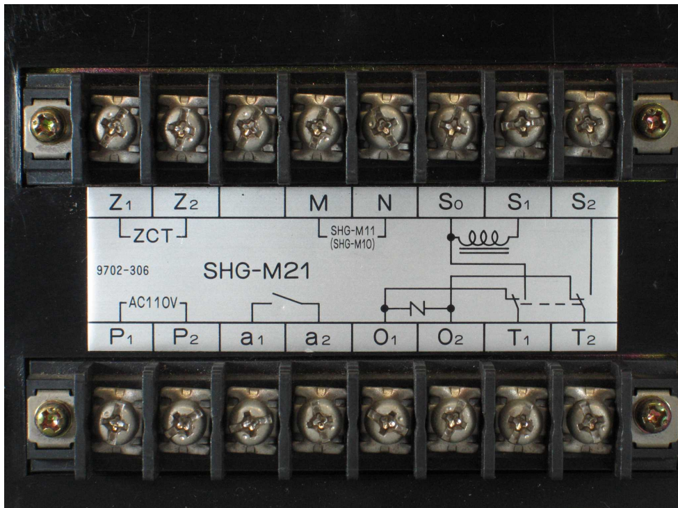
SHG - M21 端子配列
