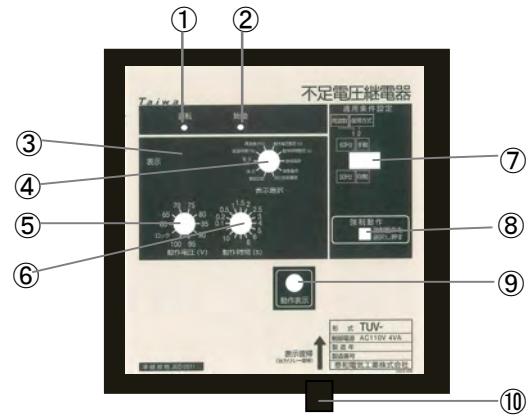
図6 TUV-DV10 正面図
