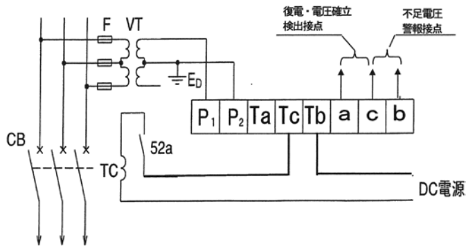
図5 外部接続図 (例)
