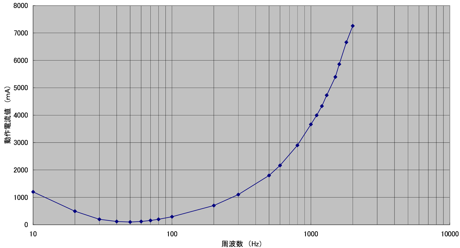
漏電継電器 LL-30K の周波数特性 50Hz 100mA整定
