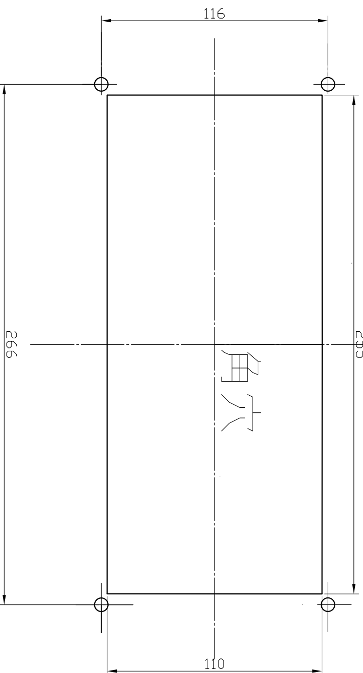
パネルカット寸法
