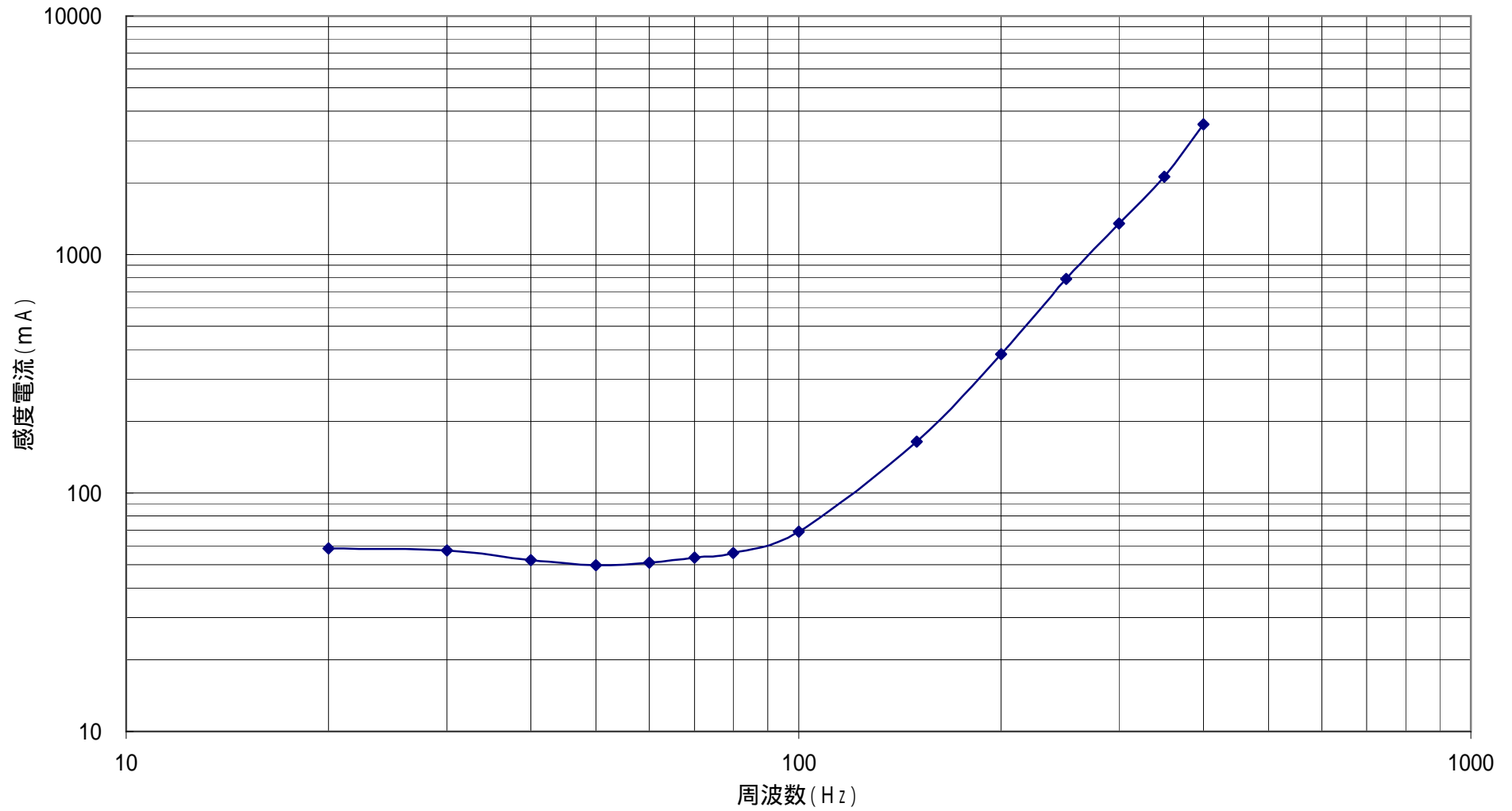
LGF - 51F周波数特性 I o 計測値 = 50mAとなる1次電流値
