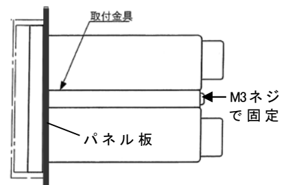
図2 取付状態図
