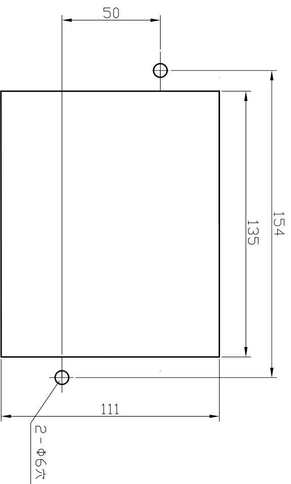
取付け穴加工図
