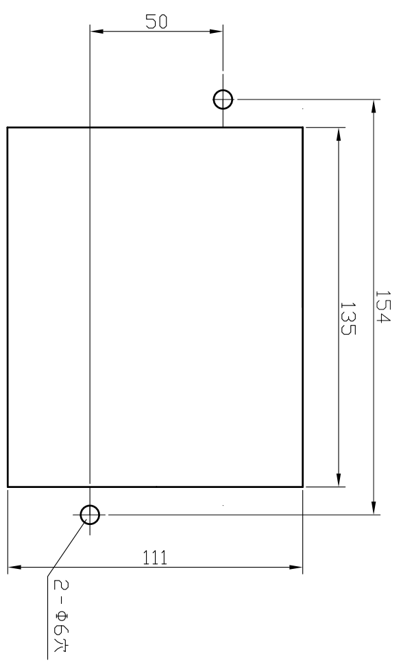
取付け穴加工図
